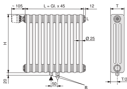
Встроенный вентиль вверх, подключение внизу по центру 1)
