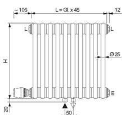
2-трубное подключение, нижнее, центральное
